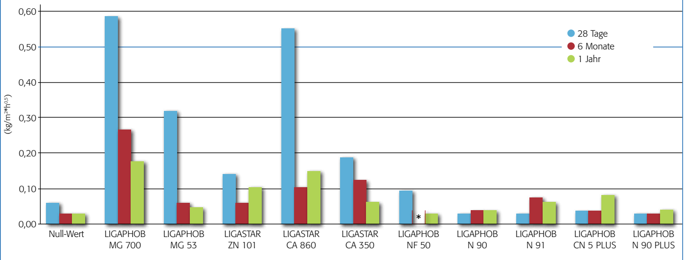
Abb. 5: Wasseraufnahmekoeffizient
